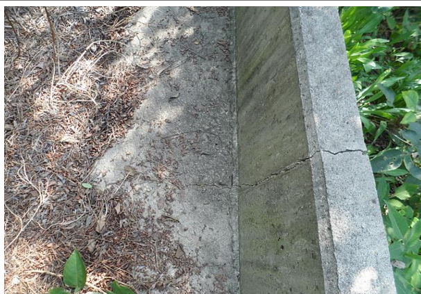
소단 배수로 균열
